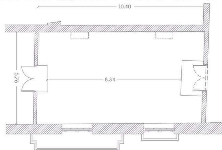
Planta 1ª
